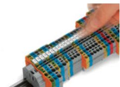
Naklapnutí štítků WMB Inline do držáků značení.
