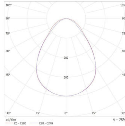
KANLUX S.A. (kat 37271) BLINGO U E125LM 30NW / Krzywa rozsytu światła (biegunowo)
