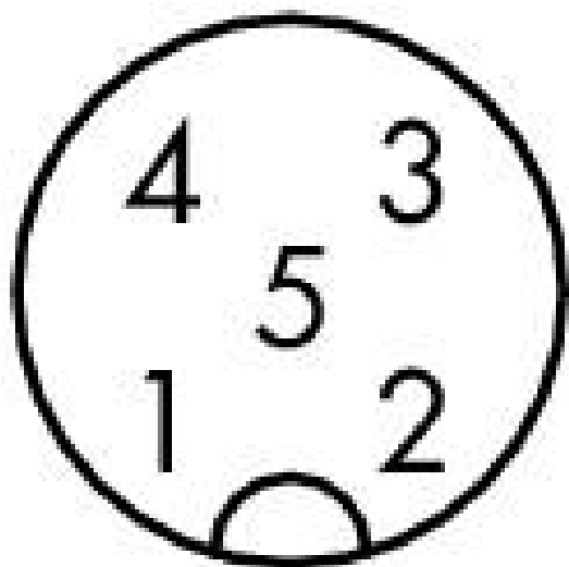
M12-Stecker
