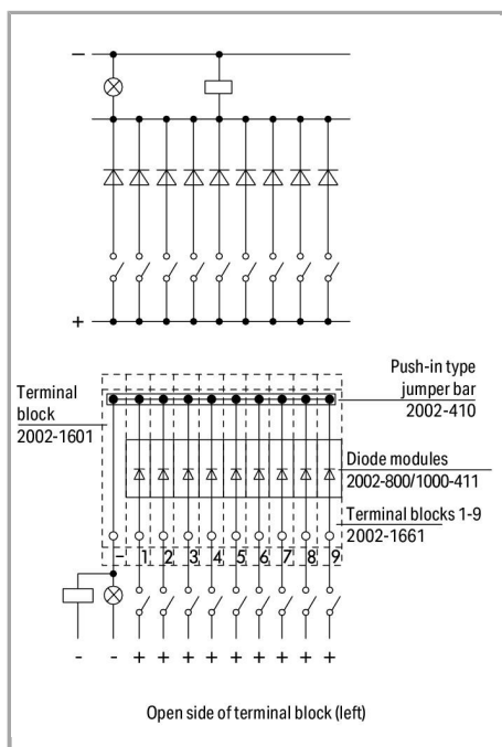
Diode module (2002-800/1000-411)
