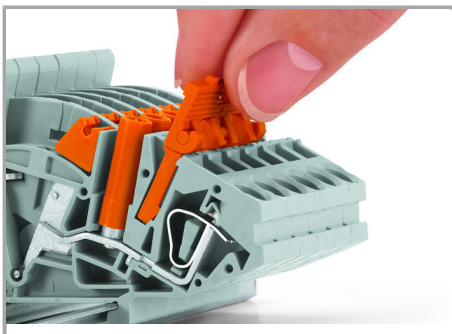
Změny vyhrazeny. Removing a jumper via safety lid.
