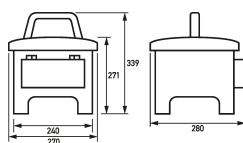
Maßzeichnung Gruppenansicht
